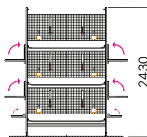
3 tiers
