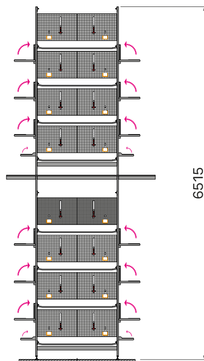
8 tiers DD
