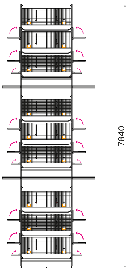
9 tiers TD
