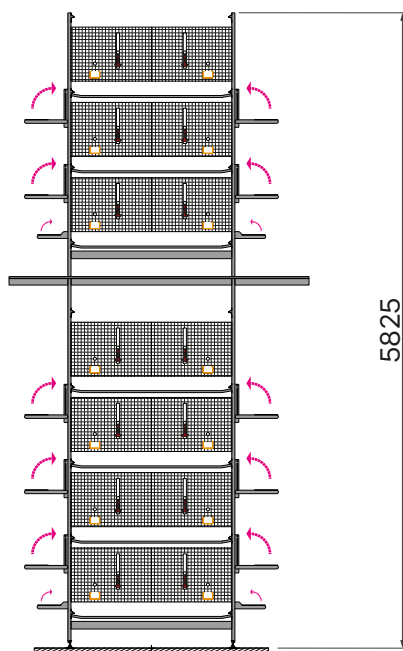
7 tiers DD
