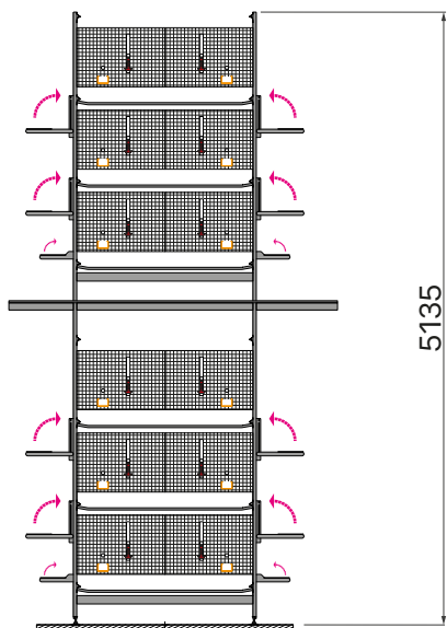
6 tiers DD
