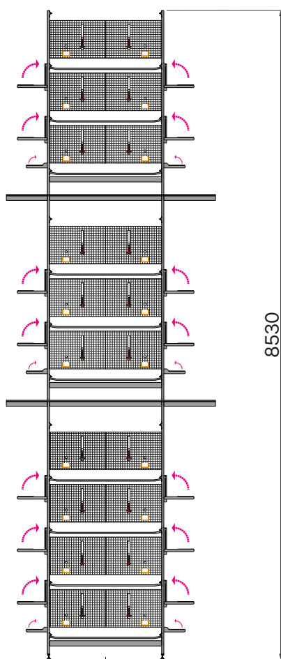
10 tiers TD
